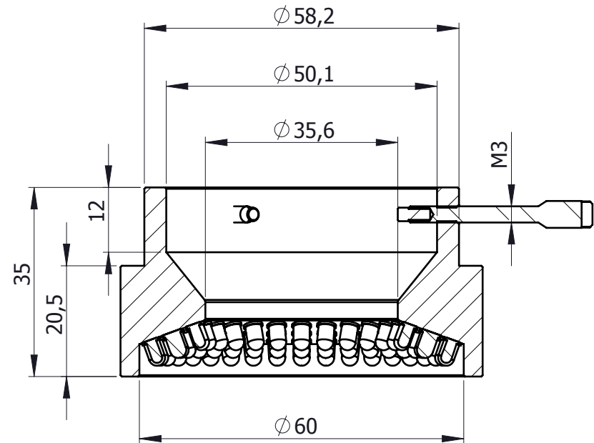
SCHNITT A-A
